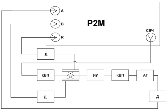
Д — детектор, КВП — коаксиально-волноводный переход, АТ — аттенуатор, ИУ — измеряемое устройство
