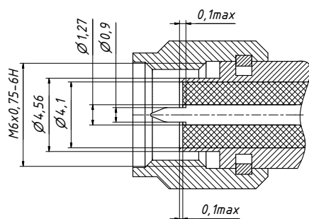
Соединитель тип IX, вар. 1 (вилка)
