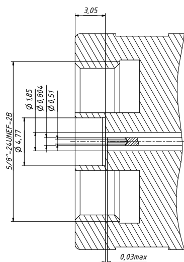
Соединитель тип NMD 1,85 мм (розетка)
