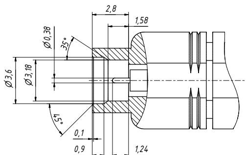
Соединитель тип SMP (вилка, smooth bore)
