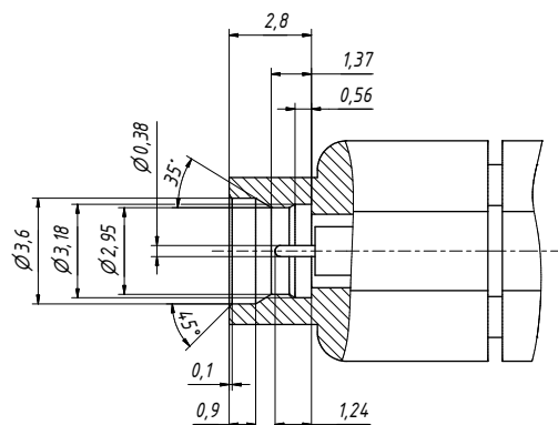
Соединитель тип SMP (вилка, full detent)
