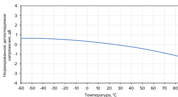
Зависимость детектируемого напряжения, нормированного относительно температуры 25 °С, от температуры окружающей среды (при входной мощности 10 дБм и частоте 1 ГГц, R_n = 30 \text{ кОм} )
