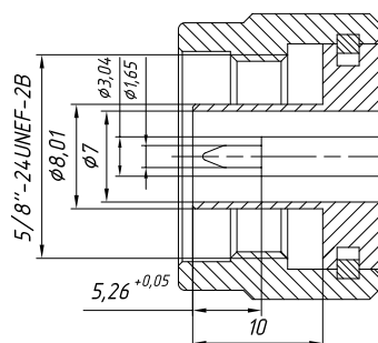
Соединитель тип N (вилка)
