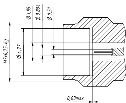
Соединитель тип 1,85 мм (розетка)
