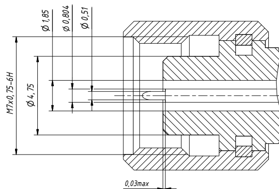
Соединитель тип 1,85 мм (вилка)
