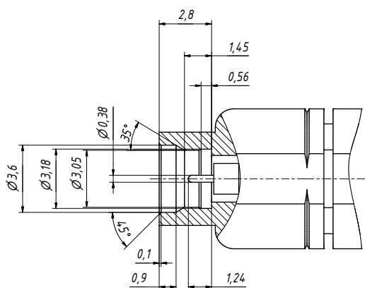
Соединитель тип SMP (вилка, limited detent)
