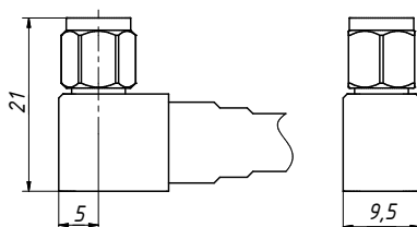
Тип IX вар.3 (вилка) для серии KC20A2Y и KC20A2Y Тип 3,5 мм (вилка) для серии KC20A2Y и KC20A2Y
