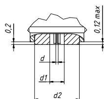
Присоединительные размеры ПКМ2 с приборной стороны
