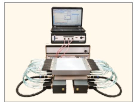
Рис. 8. Внешний вид комплекса K2M-102, скоммутированного для калибровки
