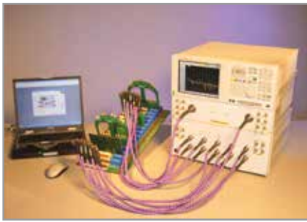
Рис. 2. Измерительный комплекс Agilent U3025AE10
