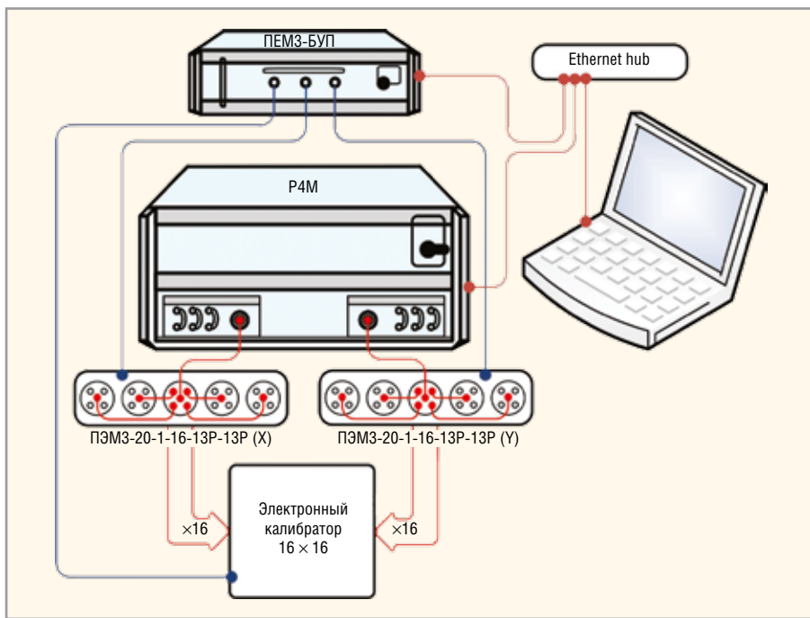
Рис. 5. Структурная схема комплекса K2M-102
