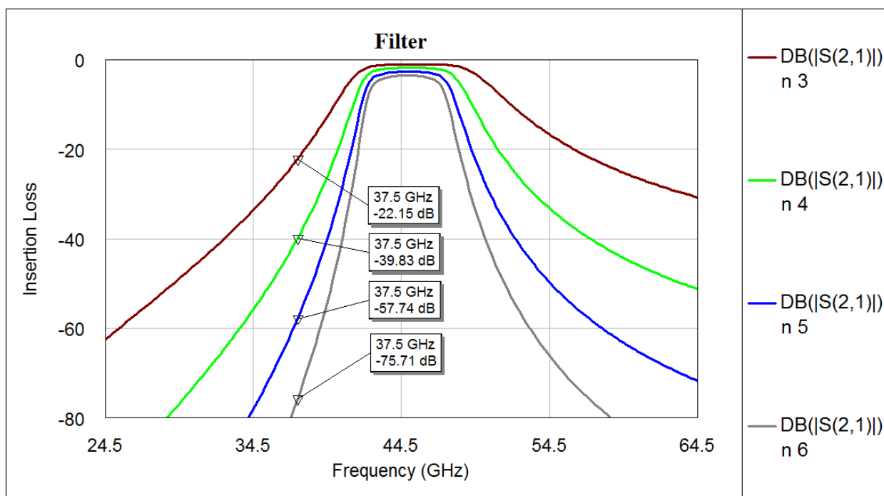
Рис. 1. Амплитудно-частотные характеристики ППФ с различным числом звеньев
