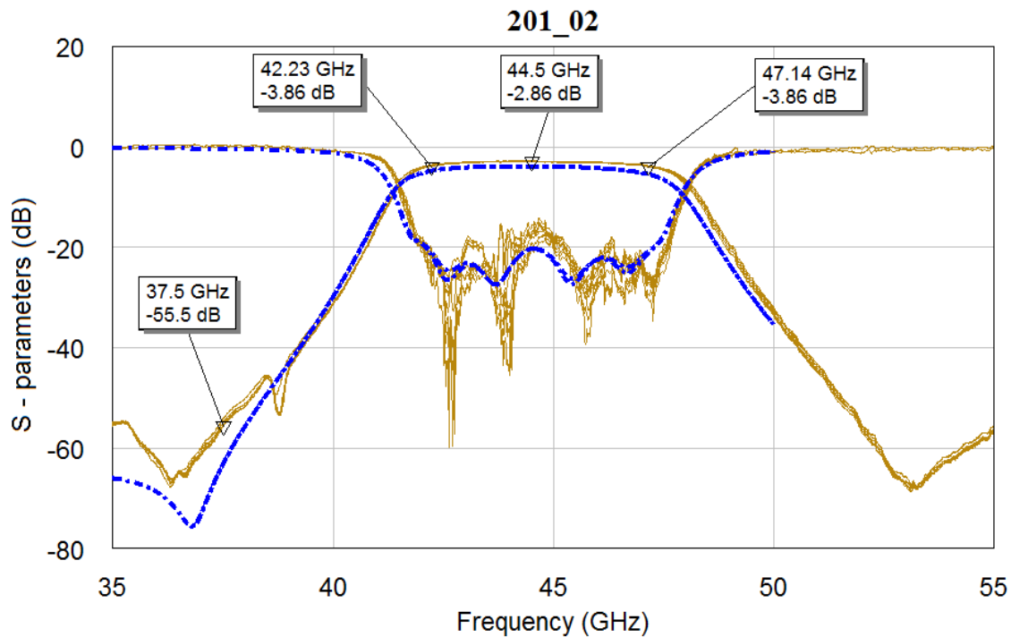
Рис. 4. Сравнение расчетных и практических характеристик: а) 5-резонаторный фильтр MQ 201-01 б) 6-резонаторный фильтр MQ201-02
