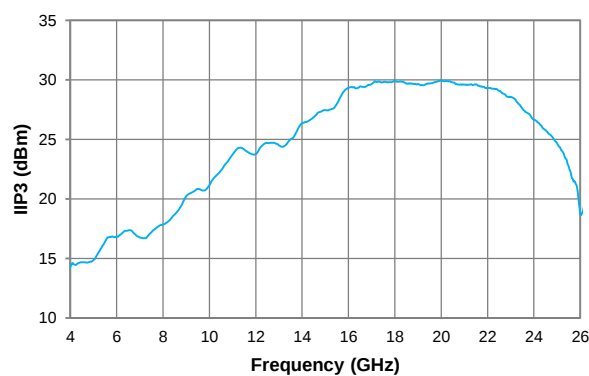
Input IP3
