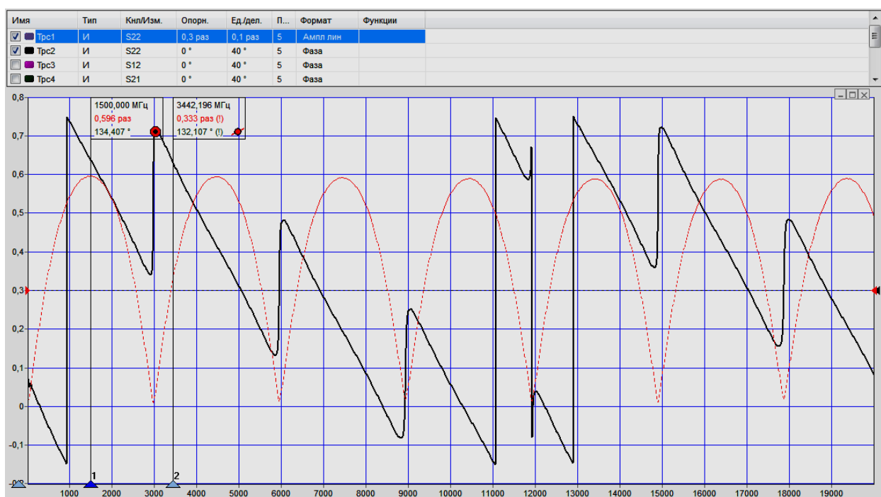
Рисунок 13 – Типичная фаза коэффициента отражения (S22) воздушной линии 25 Ом
