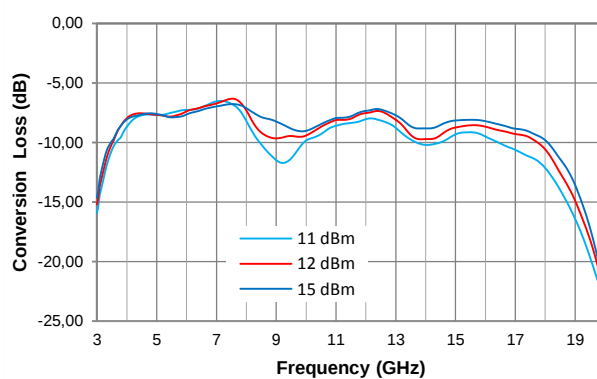
Conversion Loss (config. B)
