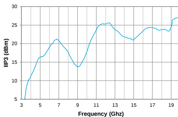
IIP3 (config. B)
