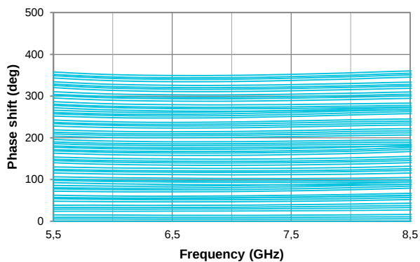
Phase shift
