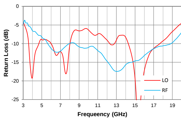
Return Loss (config. A)
