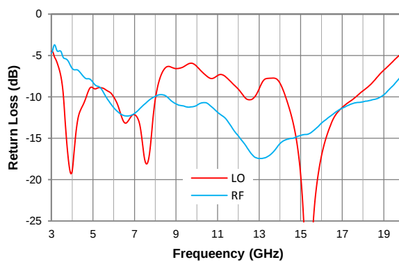
Return Loss (config. B)
