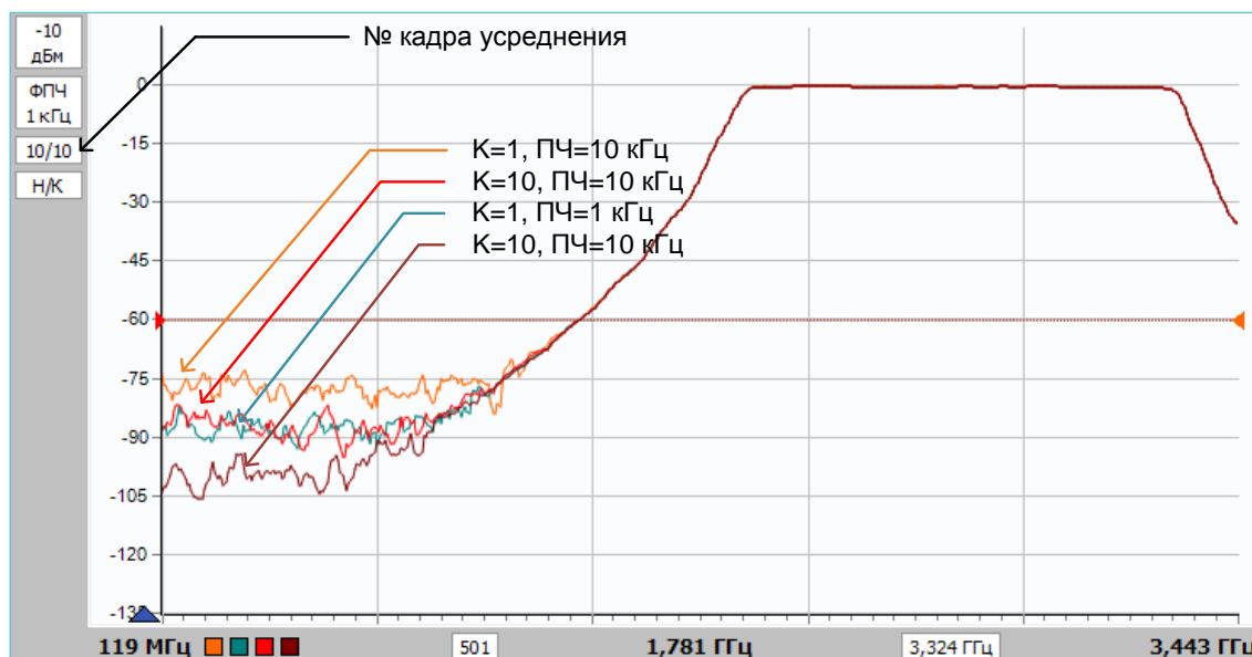
Рисунок 5.2 – Влияние усреднения и полосы пропускания фильтра ПЧ
