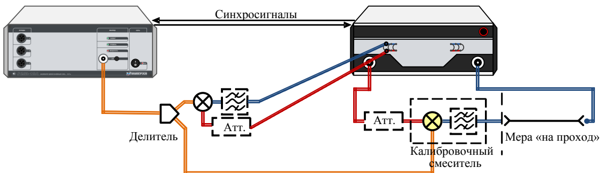
Рисунок 5.36 – Схема измерения параметров передачи «калибровочного» смесителя (шаг 10)
