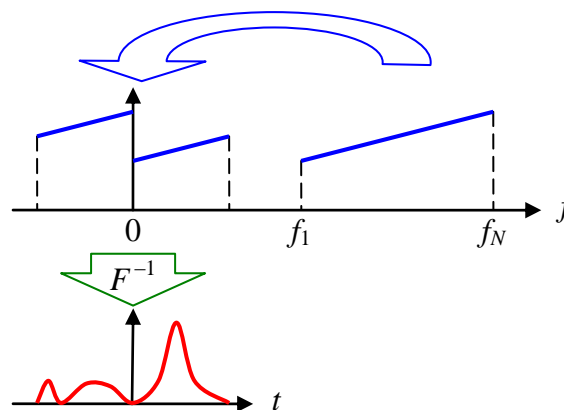
Рисунок 5.14 – Преобразование BandPass
